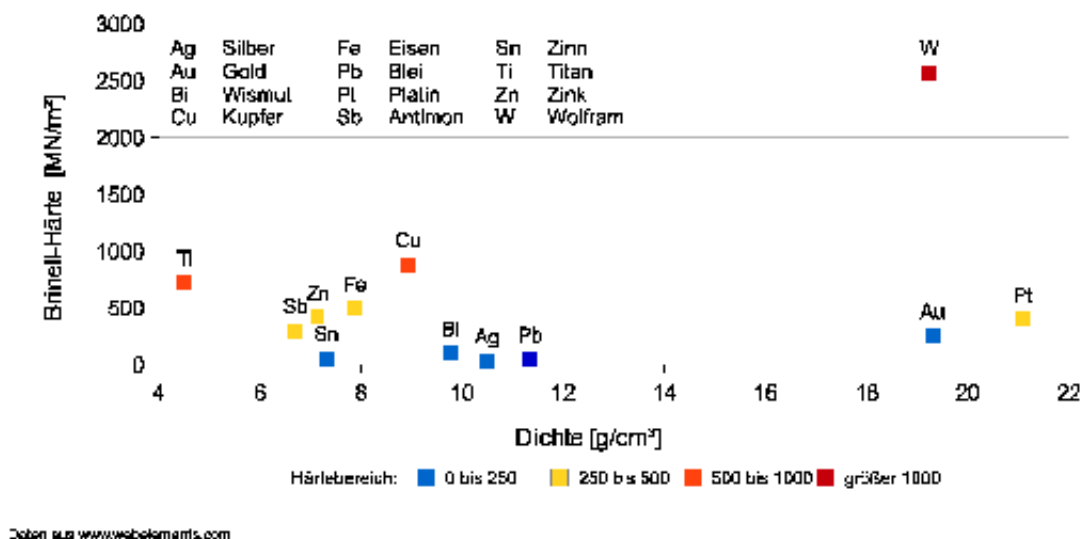
Abb.1: Vergleich der Dichte und Brinell-Härte von Alternativmetallen relativ zu Blei (Daten aus www.webelements.com )
