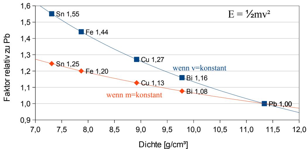
Abb. 2: Vergleich des Energietransports von Alternativmetallen relativ zu Blei
